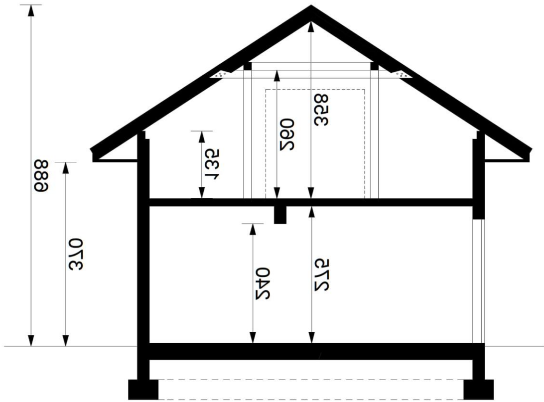
Przekroje
