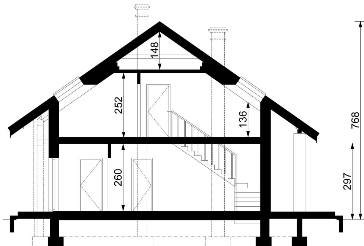
Przekroje
