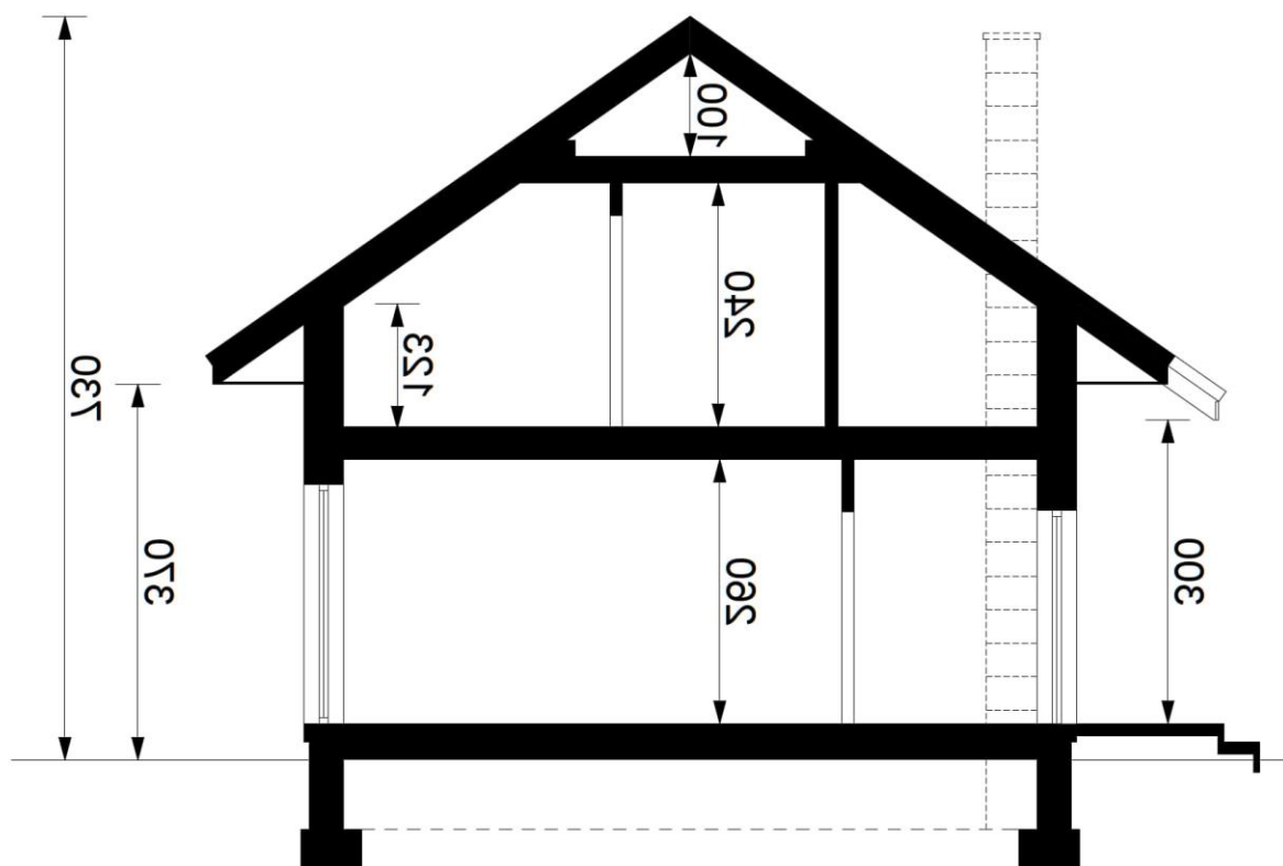
Przekroje
